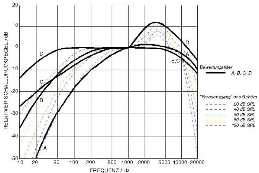
Abbildung 16: Bewertungsfiler A, B, C und D und Frequenzgang des Gehörs
