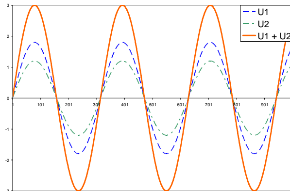
Abbildung 4: Addition zweier korrelierter Spannungen, Phasenwinkel 0^\circ Blau ist Spannung U_1 , Grün Spannung U_2 , Rot die Summenspannung U
